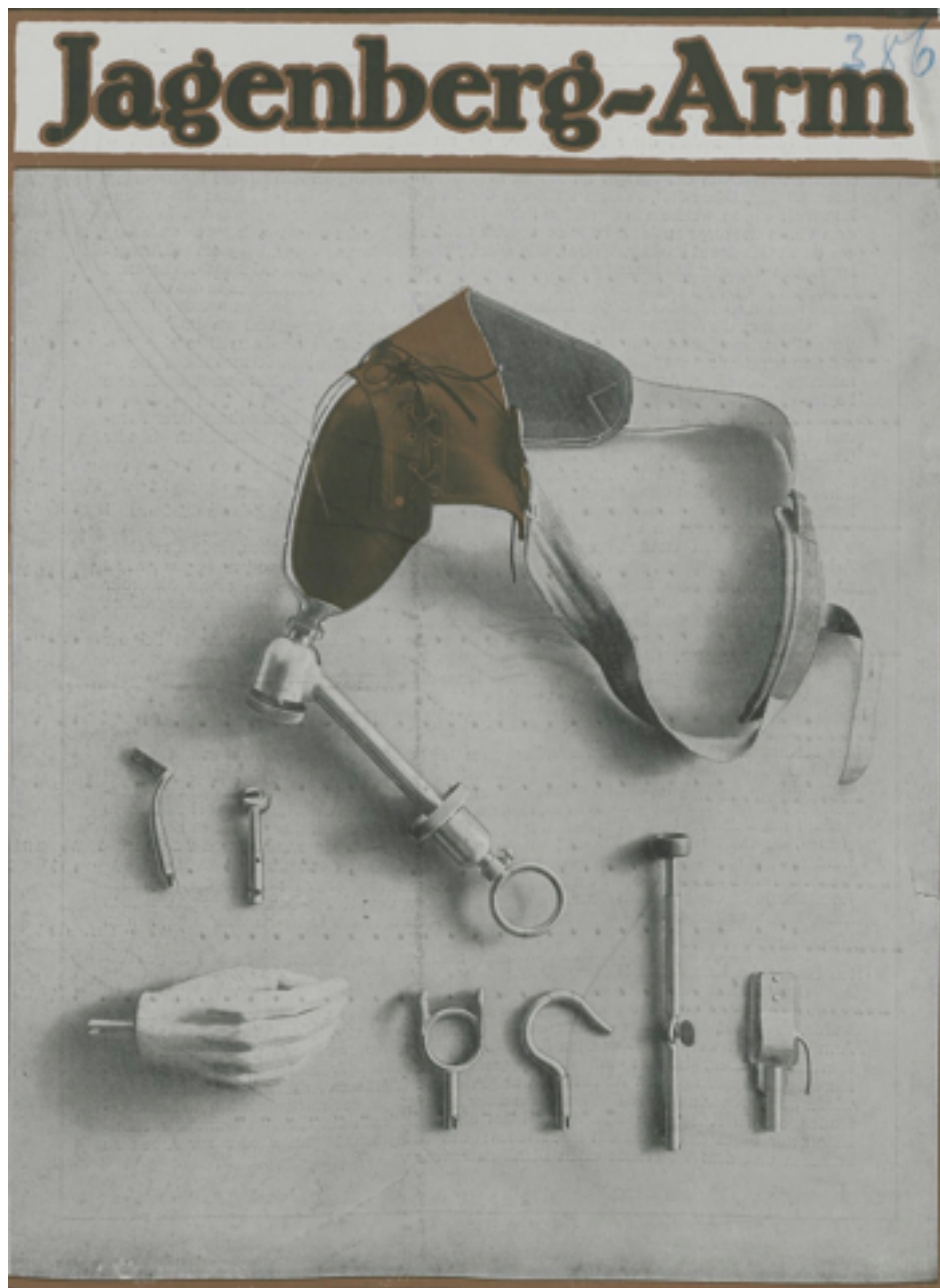
Abb.2 2 : Historische Fotografie eines Jagenberg-Arms mit verschiedenen Aufsätzen.
